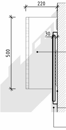
Креслення консолі з дзеркалом в плані
