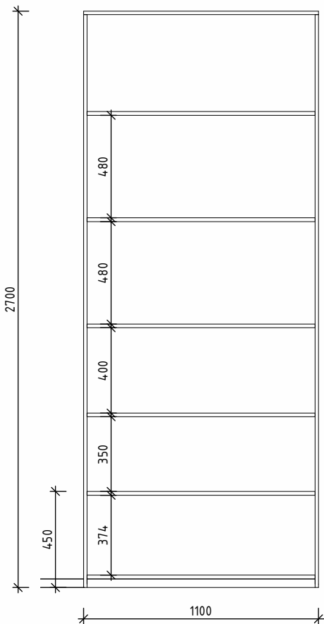
Шафа у відкритому стані
