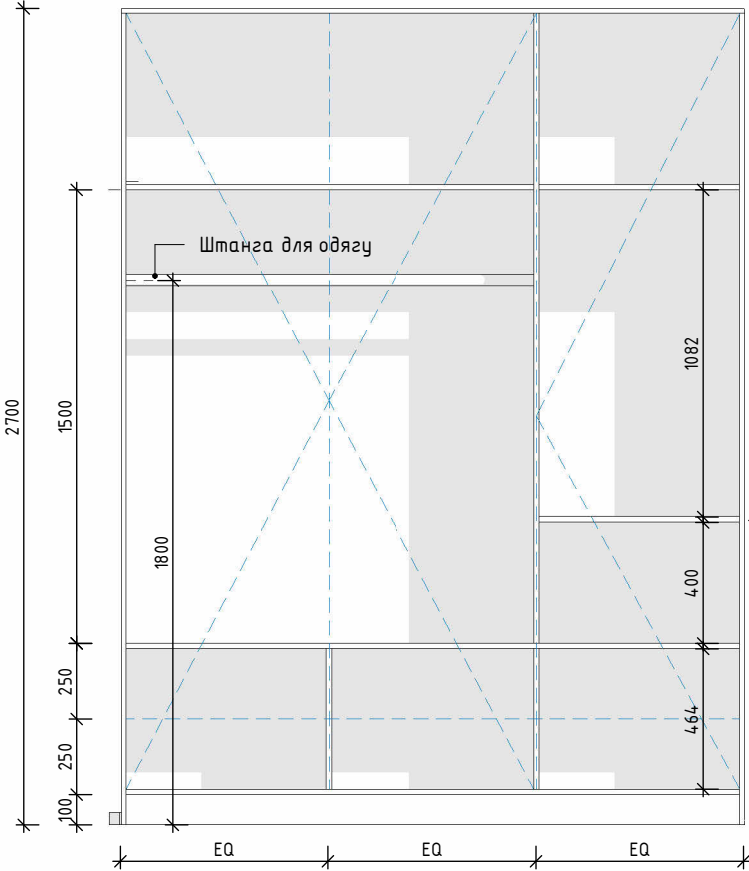
Шафа у відкритому стані
