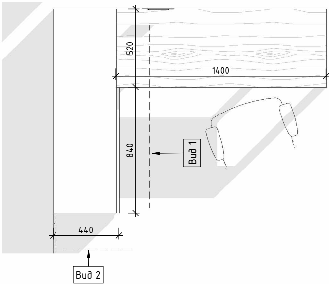
Загальні габарити в плані
