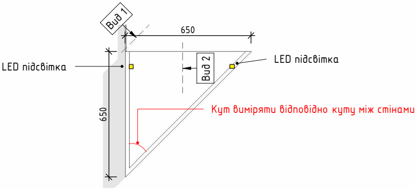
Загальні габарити в плані
