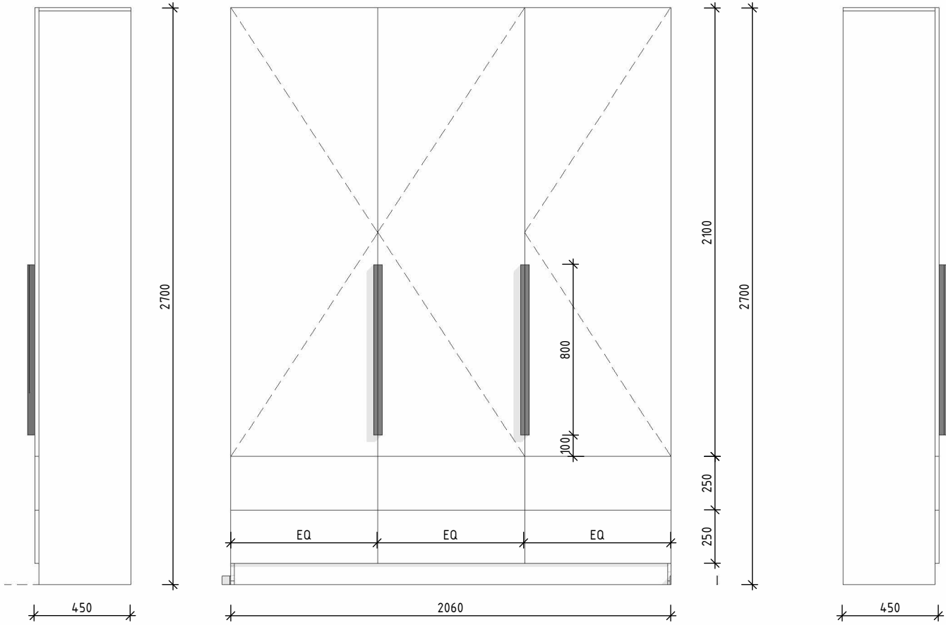
Шафа у відкритому стані
