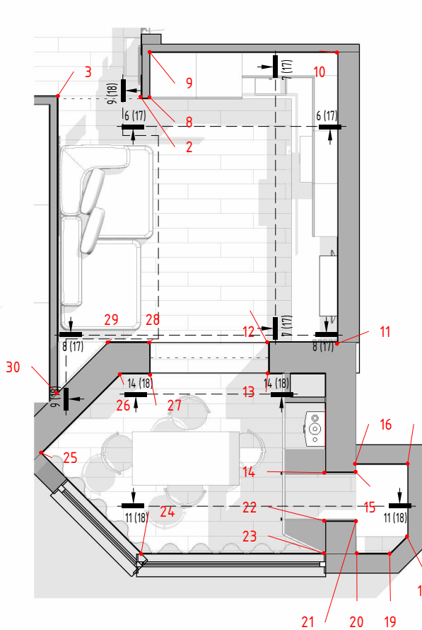
План-схема
